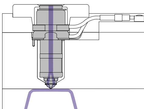
单点喷嘴直接浇注于制品
