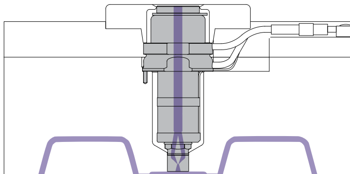
单点喷嘴直接浇注于冷流道
